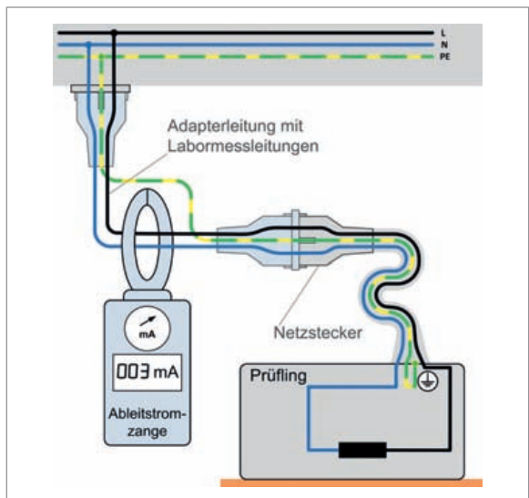
Abb. 3.13 Schutzerleiterstrom- messung mit einer Strommesszange („Leckstrommessung“)
