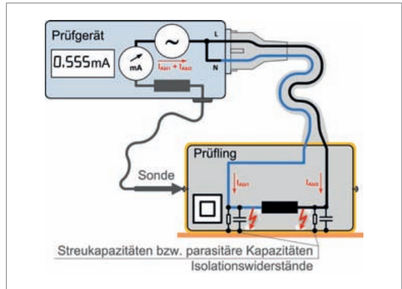
Abb. 3.18 Berührungsstrommessung nach dem Ersatz- Ableitstrommessverfahren. SK II
