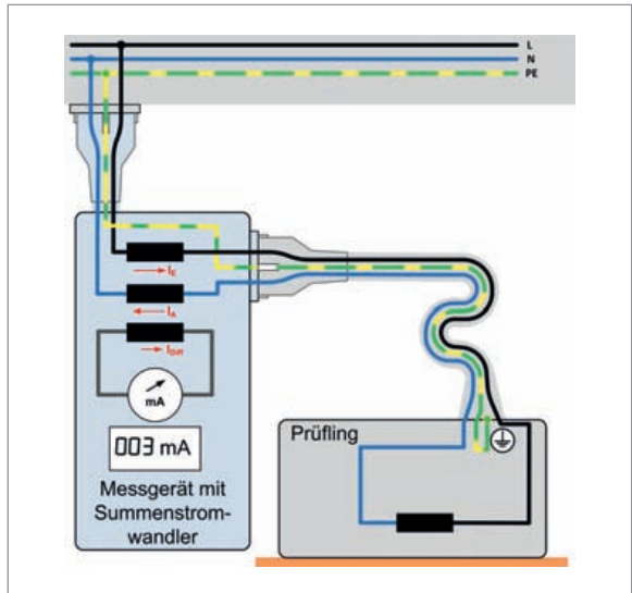
Abb. 3.12 Schutzerleiterstrom- messung nach dem Differenzstrommess- verfahren
